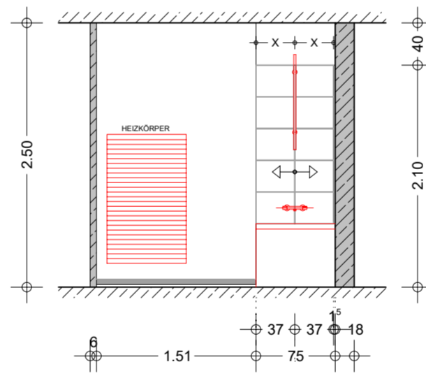
ANSICHT C - M 1:50
